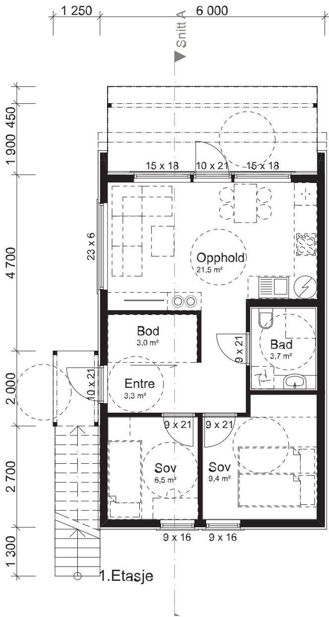
Alt 2: 4-mannsbolig, BRA 50 m 2
