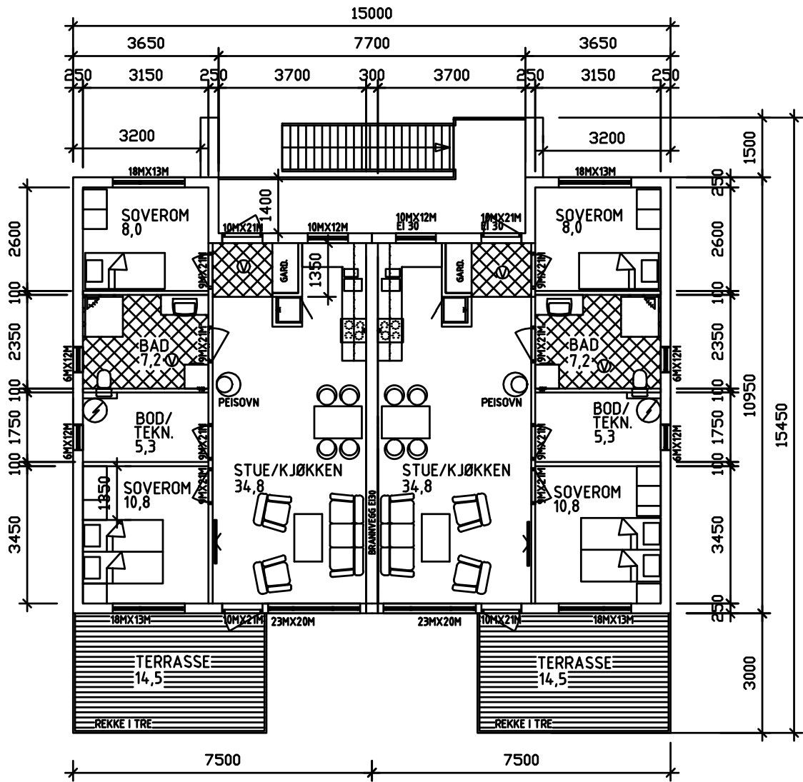
Alt 3: 4-mannsbolig, BRA 68 m 2
