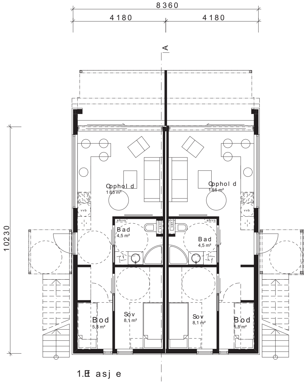
Alt 1: 4-mannsbolig, BRA 37 m²
